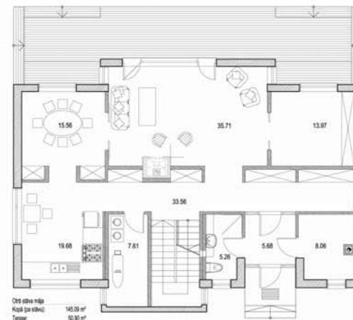
Lielā sala 1. stāva plāns
